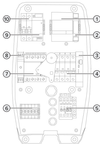
Abb. 5: Innenansicht (Beispiel: AMTRON® Professional* 22)
