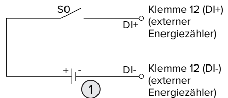
Abb. 16: Ansteuerung über ein Koppelrelais und einer zusätzlichen Spannungsversorgung
