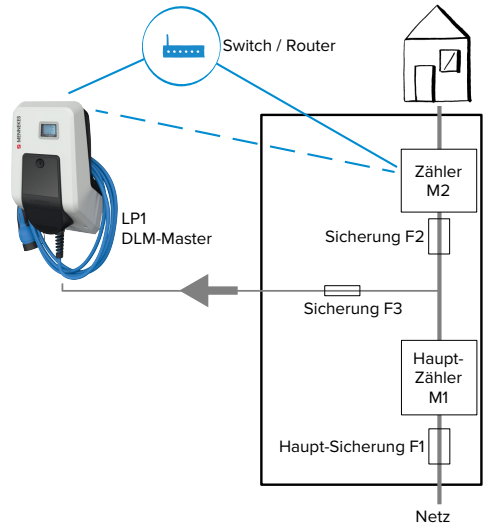
Abb. 14: Energiezähler misst nur externe Verbraucher
