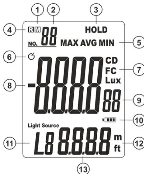
Abb. 2: Displaybeschreibung
